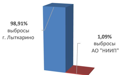
Диаграмма 10 Вклад АО «НИИП» в общий объем выбросов ВХВ г. Лыткарино
