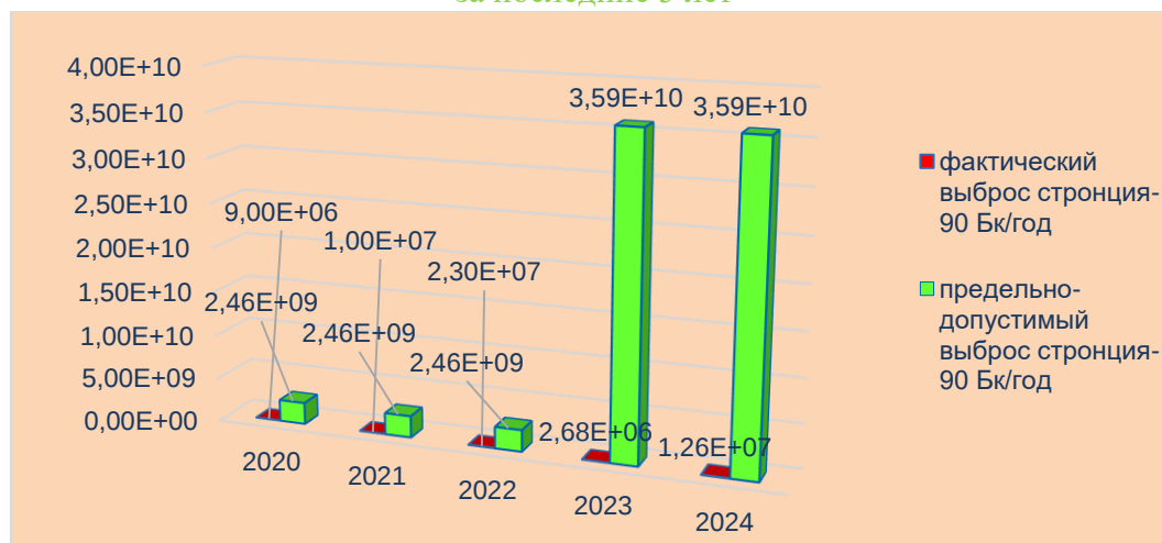
Диаграмма 7 Динамика выброса стронция -90 в атмосферный воздух за последние 5 лет
