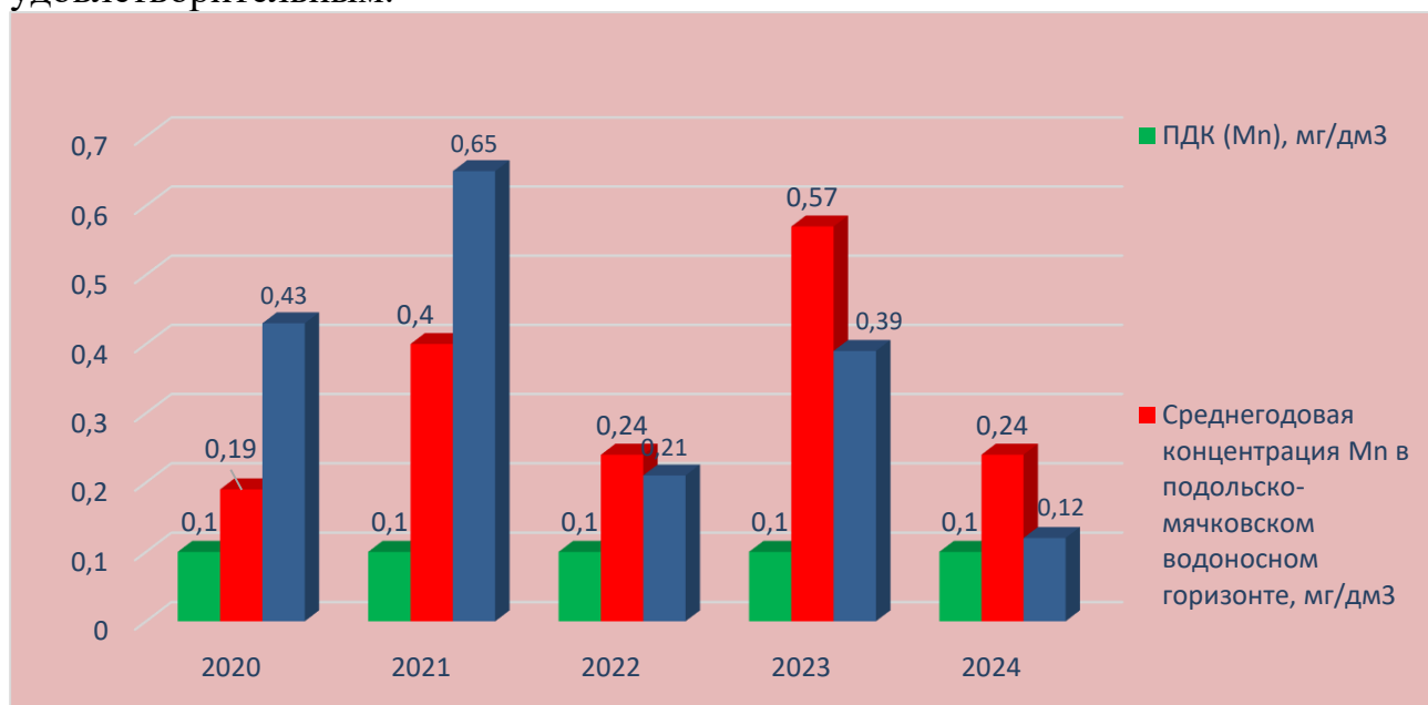
Диаграмма 1 Динамика среднегодовых концентраций марганца в подземных водах за последние 5 лет
