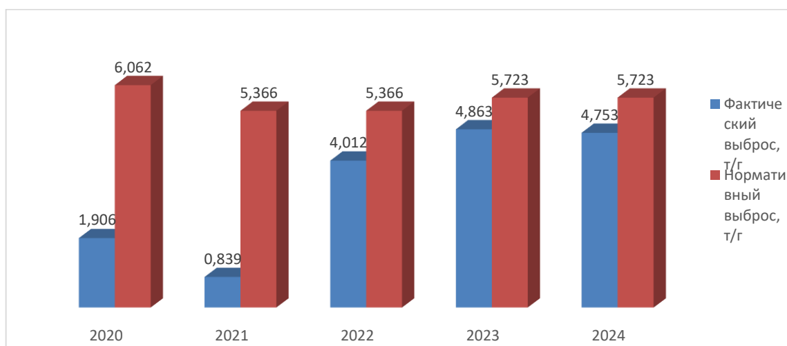
Диаграмма 5 Динамика выброса вредных химических веществ в атмосферный воздух за последние 5 лет
