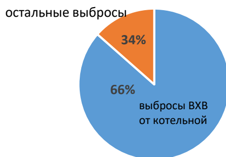
Диаграмма 4 Доля выбросов ВХВ котельной в общем выбросе предприятия
