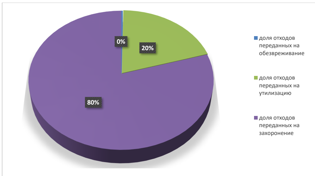
Диаграмма 9 Соотношение долей утилизированных, обезвреженных и размещенных отходов
