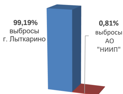
Диаграмма 10 Вклад АО «НИИП» в общий объем выбросов ВХВ г. Лыткарино
